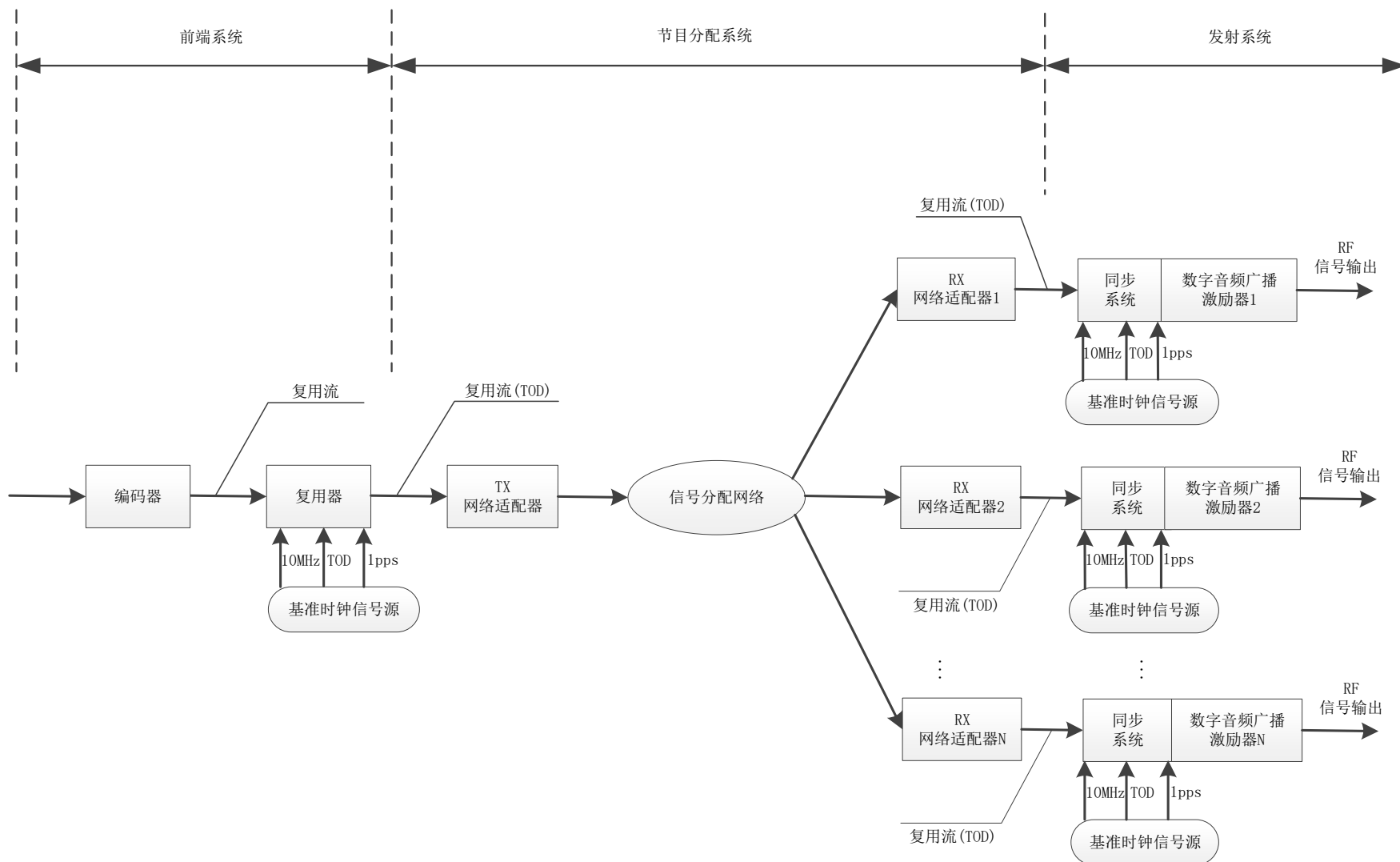
图1 调频频段数字音频广播单频网系统结构示意图
